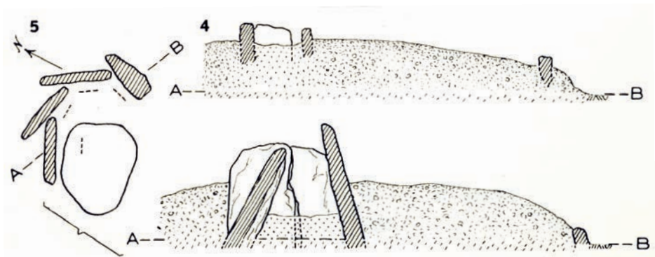
Anta 2 de S. Gens (desenhos: George e Vera Leisner, 1959)
