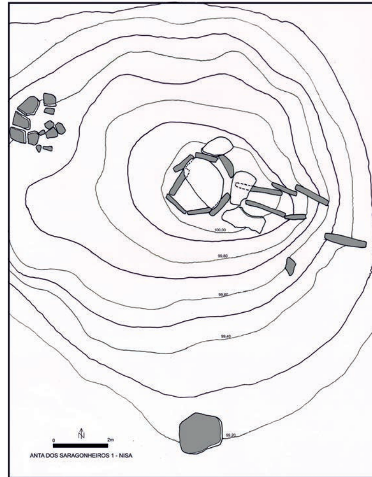
Levantamento topográfico da Anta 1 dos Saragonheiros
